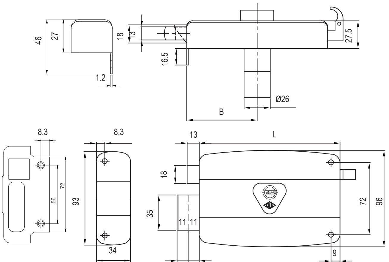
Технический чертеж двух-поворотного замка
